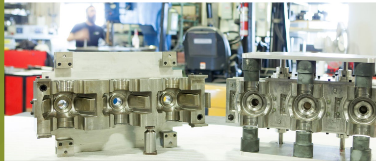
Modèles pour pièces coulées dans le sable et moule permanent.
